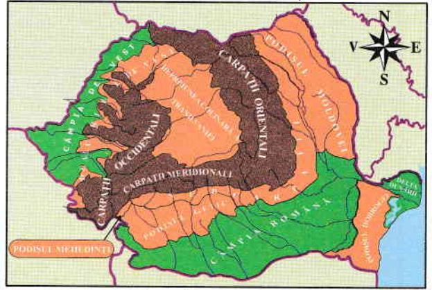
ROMÂNIA. TREPTE ȘI UNITĂȚI DE RELIEF
